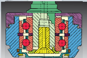
Rodamientos de cerámica a contacto oblicuo.
