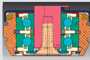
Rodamientos en cerámica lubricados manualmente.
