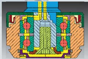
Rodamientos de cerámica lubricados durante el proceso completo de trabajo.
