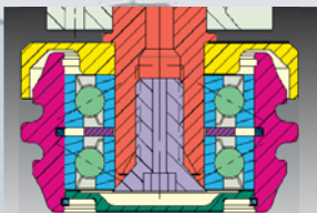
Ruedas de cierre doble perfil.
