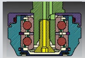
Rodamientos de cerámica lubricados durante el proceso completo de trabajo y junta en espiral.
