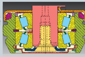
Rodamientos cónicos lubricados manualmente.
