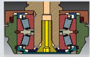
Rodamientos cónicos lubricados durante el proceso completo de trabajo y junta en espiral.
