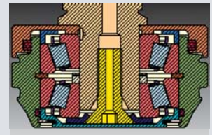
Cuscinetti a rulli conici con lubrificazione a ricircolo e tenuta a spirale.
