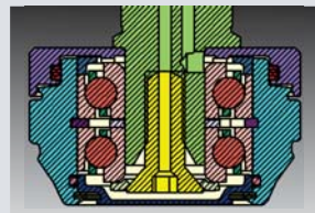
Cuscinetti in ceramica con lubrificazione a ricircolo e tenuta a spirale.
