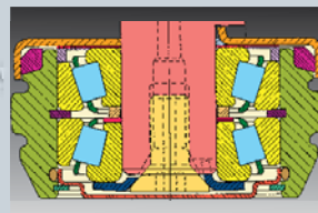
Cuscinetti a rulli conici con lubrificazione manuale.
