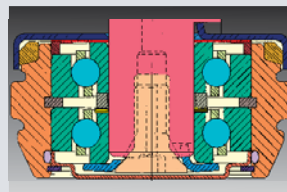
Cuscinetti in ceramica con lubrificazione manuale.
