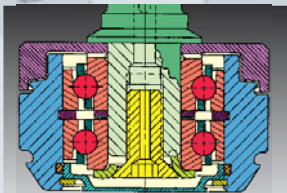
Cuscinetti in ceramica a contatto obliquo.
