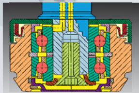
Cuscinetti in ceramica con lubrificazione a ricircolo.
