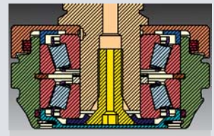
Automatische Schmierung mit Kegelrollenlagern und Labyrinthdichtung
