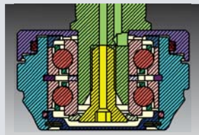
Automatische Schmierung mit Keramik-Kugellagern und Labyrinthdichtung
