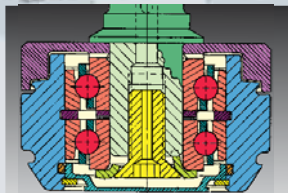
Schulterlager mit Keramik-Kugellager
