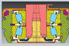
Manuelle Schmierung mit Kegelrollenlager
