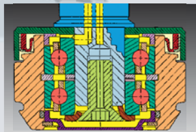
Manuelle Schmierung mit Keramik-Kugellager
