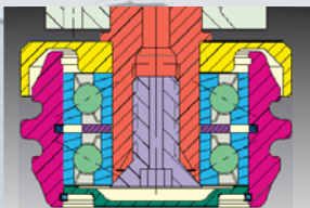
Molettes de sertissage à cannelure double
