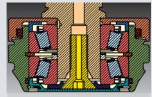
Lubrification interne avec rouleau conique et étanchéité par labyrinthe
