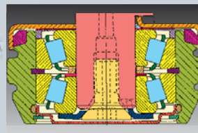
Pas de lubrification interne avec rouleau conique
